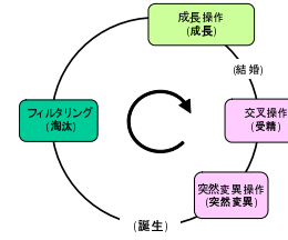
図 6 粒子フィルタと遺伝的アルゴリズムの類似性．一般状態空間モデルの R_t(y_t | x_t) を GA での目的関数に読み替えるだけで，アルゴリズムの構成は GA と粒子フィルタはほぼ同じである．特にフィルタの手続きは，GA での淘汰の手続きと全く同じである．また，予測の手続きは，システムモデルにおいて確率的な揺らぎを導入するという意味においては，GA の突然変異と交叉の確率的操作に対応する． F_t による粒子フィルタでの非線形状態更新操作（図では成長操作と呼んでいる）は GA にはない．
