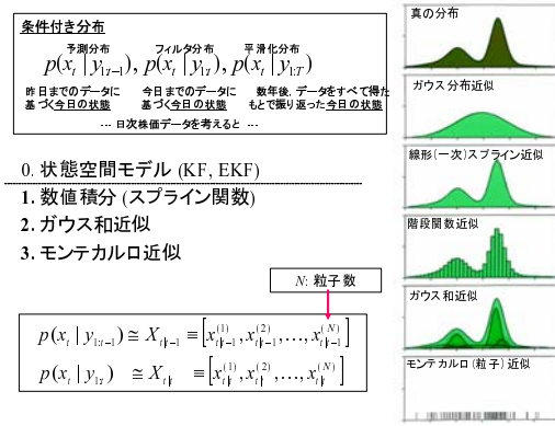
図 3 条件付き分布とその近似表現法。一般状態空間モデルに関連する重要な問題は、予測、フィルタおよび平滑化の 3 つの条件付き分布 (周辺分布) の計算に帰着できる。一般に条件付き分布は非ガウス分布となるので、その分布表現に何らかの形での近似が必要である。粒子フィルタは究極の近似、つまり多数の実現値 (粒子) によるモンテカルロ近似に基づく。番号 (0-3) が増えるほど、高次元分布の表現が省力的かつ柔軟になる。
