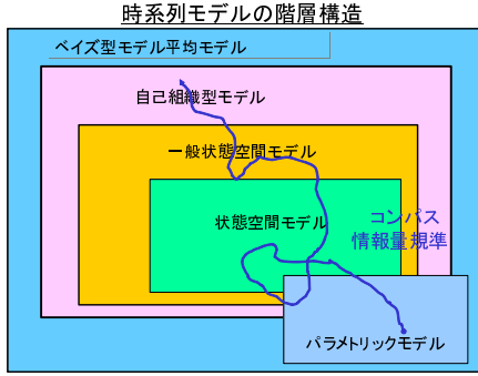
図1 時系列モデルの高度化。線形・ガウスモデルである状態空間モデルは、制御、非定常時系列解析、信号処理などの幅広い分野で使われている、基盤の時系列モデルである。有名なカルマンフィルタは状態空間モデル用の効率良い計算アルゴリズムである。広範囲の時系列モデルが、状態空間モデルの一般化版である。一般状態空間モデルと呼ばれるモデルで表現できる。カオス時系列モデルも、もちろん表現できる。また隠れマルコフモデルは状態値、観測値ともに離散値のみ許される一般状態空間モデルの特殊なケースである。シミュレーション科学と統計科学の融合技術であるデータ同化手法も、一般状態空間モデルの枠組みで議論できる。一般状態空間モデルは、メタなパラメータの時間変化も取り扱える自己組織型時系列モデルや、モデル切り替え、モデル統合なども可能にするモデル平均時系列モデルへと拡張発展している。なお、情報量規準（用語）を採用することで、より良いモデルの選択が一貫して可能である。つまり情報量規準はモデル群の海原のコンパスの役割を果たす。
