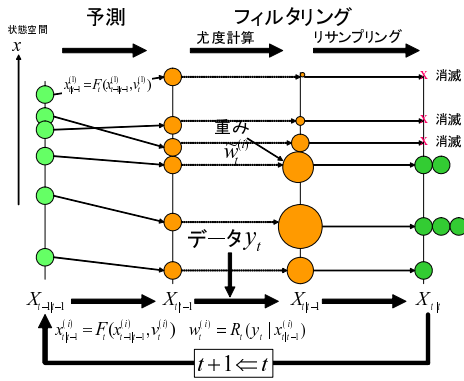
図 5 粒子フィルタアルゴリズムの概略図．時刻 t-1 の各フィルタ粒子 x_{t-1}^{(i)} に対して，ノイズ分布 q(v) から発生したシステムノイズボール v_t^{(i)} をぶつけ，非線形発展方程式 F_t でもって状態を更新する．得られた予測粒子 x_{t|t-1}^{(i)} の時刻 t のデータへの適合度，つまり各粒子の尤度（質量と思えば以降わかりやすい）を R_t(y_t | x_{t|t-1}^{(i)}) でもって評価する．各粒子の尤度を集団の尤度（ = W_t ）で規格化した確率 \tilde{w}_t^{(i)} で予測粒子をリサンプリングする．得られた粒子が時刻 t のフィルタ粒子となる．粒子フィルタではフィルタリングの操作終了後，各粒子の出現確率を等しくしている（質量を同じにする）ので，リサンプリングが必要となる．適合度が悪いと図にあるように死滅する可能性が高い．一方適合度が高いと分裂して仲間を増やす．この操作を繰り返すのが粒子フィルタである．
