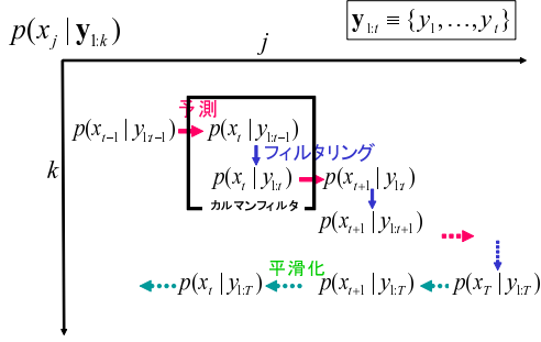
図 4 状態推定のための漸化式の模式図．右の矢印が予測の，また下矢印がフィルタリングの各操作に対応する．この操作を繰り返していけば，一番右下の p(x_T | y_{1:T}) が求まり，ここまで計算すれば左矢印の平滑化の操作により後ろ向きに逐次的に平滑化分布を求めることができる．
